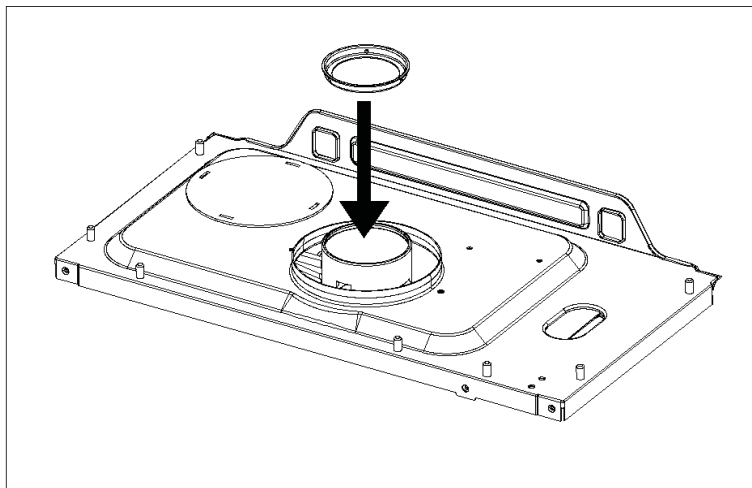
Схема установки ограничительного кольца рис.12
